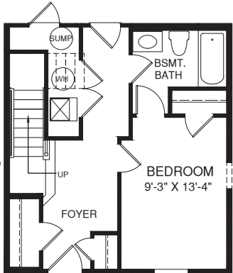
OPT. BEDROOM
